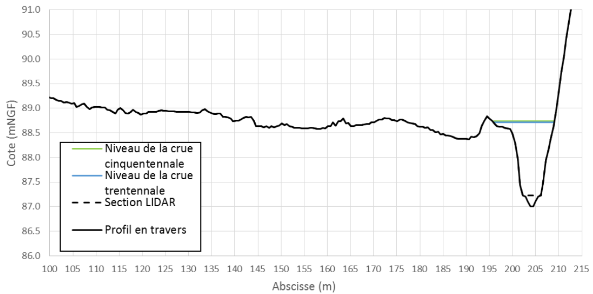
Profil en travers C - Gare de St-Pol-sur-Ternoise
