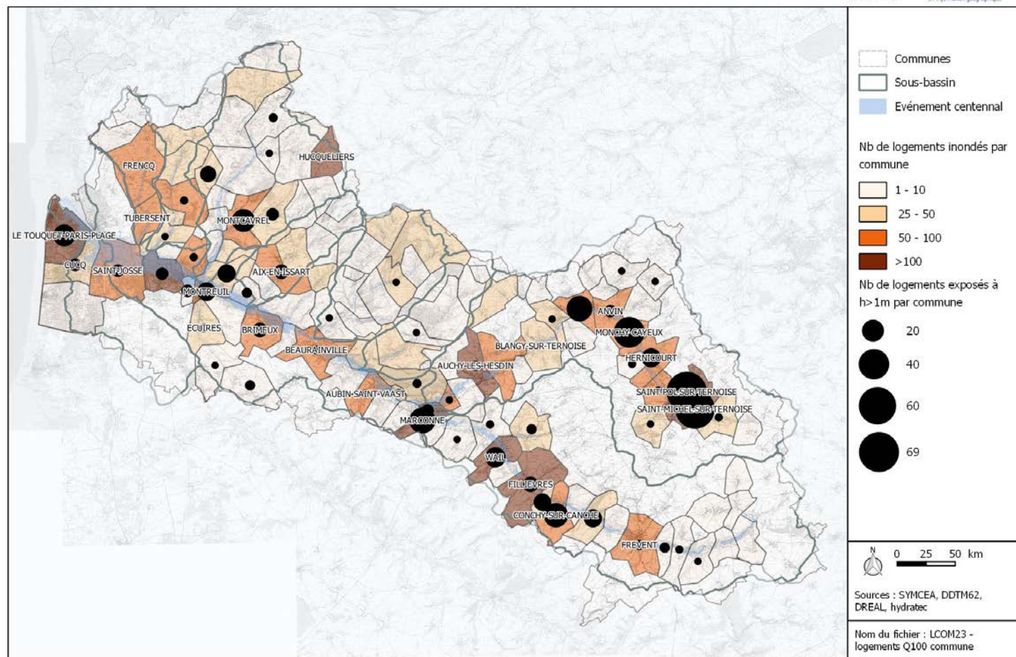
Figure 3-2 : Synthèse des principaux enjeux touchés pour une crue moyenne - Analyse du nombre d'habitations
