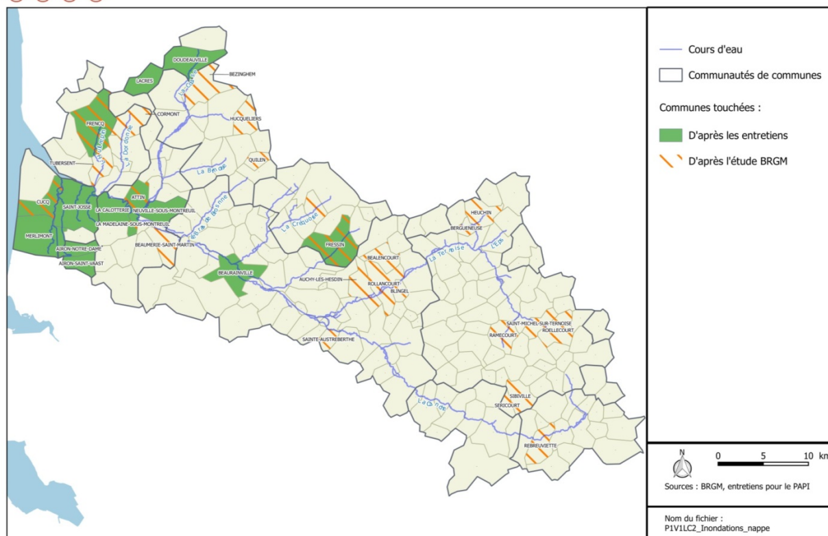
Figure 2-4 : Communes touchées par les inondations par remontée de nappe
