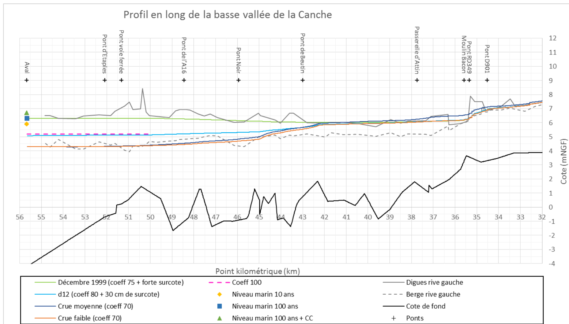
Figure 2-6 : Profil en long de la basse vallée de la Canche
