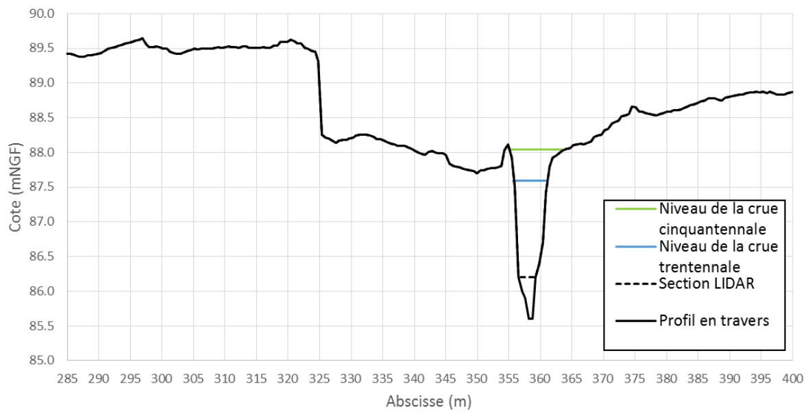
Profil en travers C - Gare de St-Pol-sur-Ternoise
