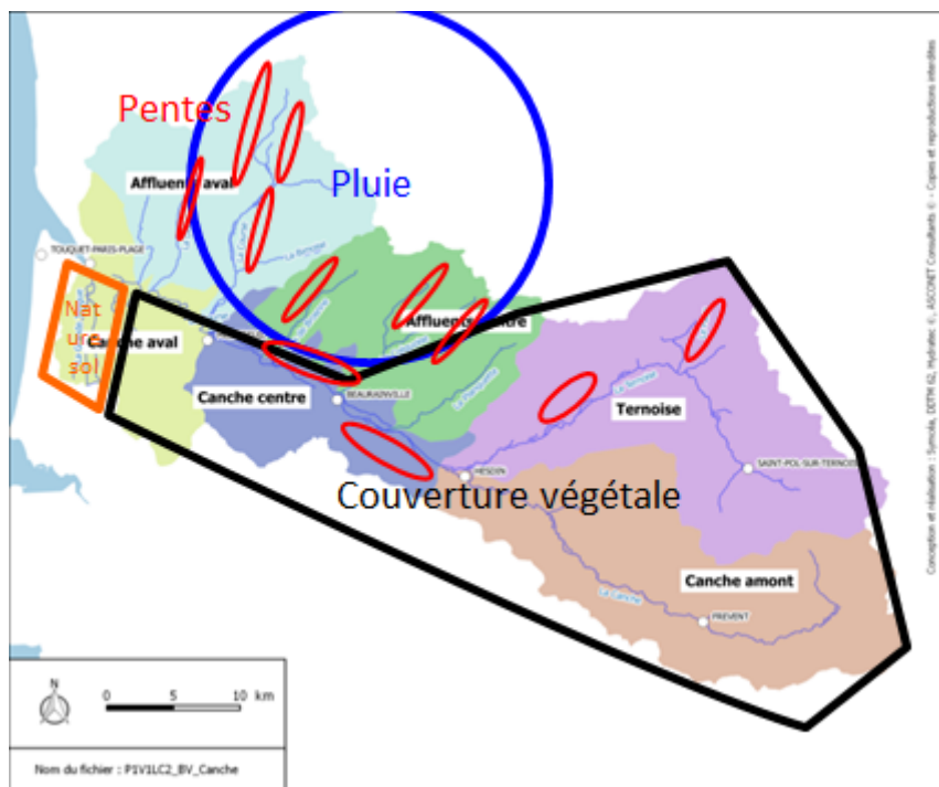
Figure 2-3 : Localisation des facteurs propices aux ruissellements
