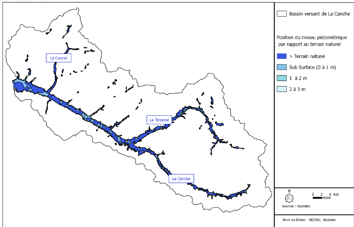
Figure 2-5: Cartographie générale des inondations par remontée de nappe sur le bassin de La Canche en période de hautes eaux (2001)
